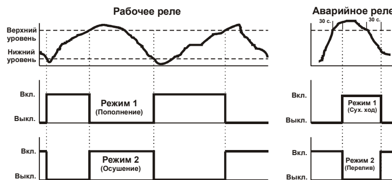
Рис.1. Диаграммы работы контроллера уровня.
